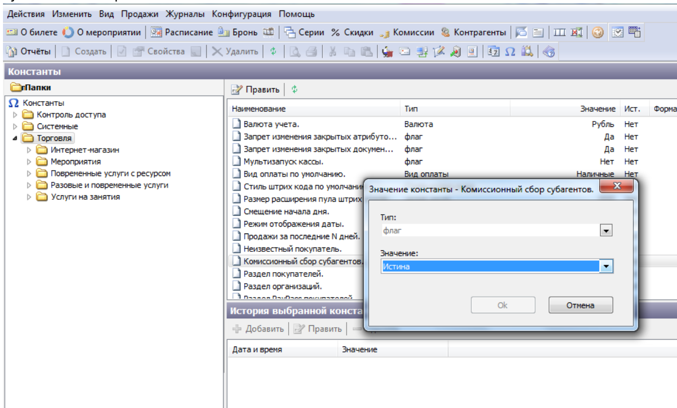
Рис.18.1. Редактирование комиссий
