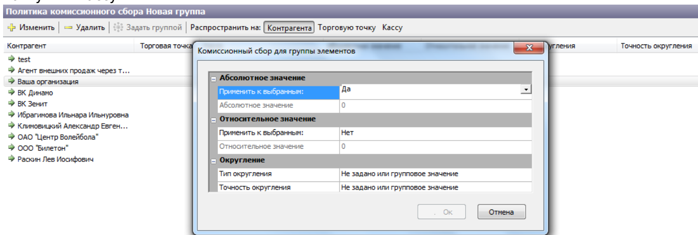
Рис. 18.2. Настойка комиссии
